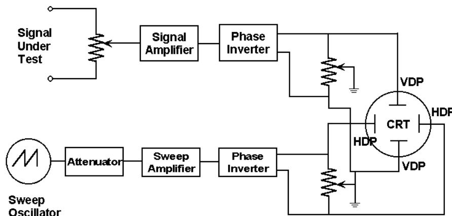
OSCILLOSCOPE
